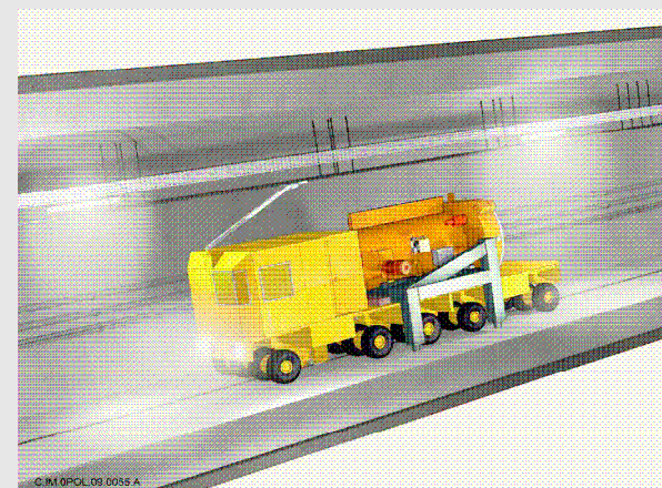
Véhicule de transfert colis HA, descenderie, image ANDRA
