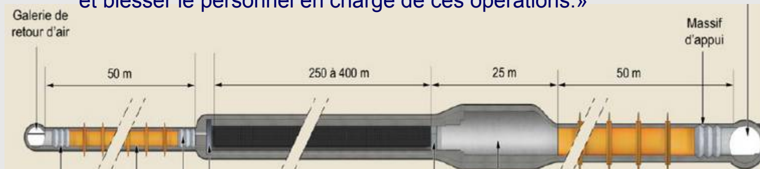
Scellement d'une alvéole MAVL, image ANDRA
