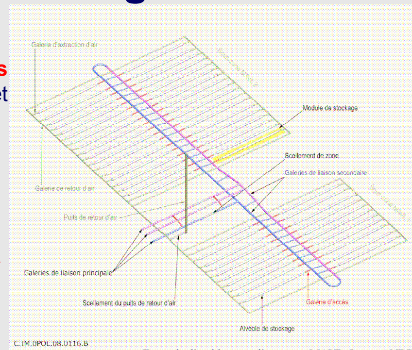
Exemple d'architecture d'une zone MAVL, Image ANDRA
